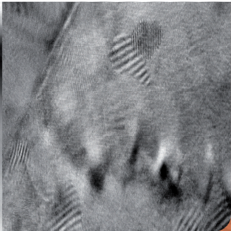
Imagem de HRTEM de contorno de grão em Nanocompósito Magnésio Nióbio processado por torção sob alta pressão (HPT). - Anderson Caires de Jesus. SENAI/MG
